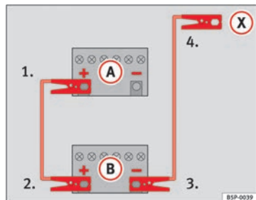
Fig. 168 Esquema para conectar los cables de emergencia en el caso de que el vehículo que suministra la corriente no disponga del sistema Start-Stop: batería descargada (A) y batería que suministra la corriente (B).
