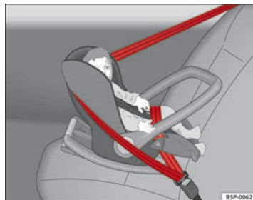
Fig. 23 Asiento para niños del grupo 0 en el asiento trasero, colocado en el sentido contrario a la dirección de la marcha.
