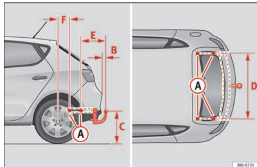
Fig. 118 Puntos de fijación del dispositivo de remolque
