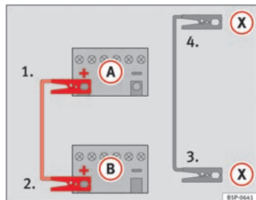
Fig. 169 Esquema para conectar los cables de emergencia en el caso de que el vehículo que suministra la corriente disponga del sistema Start-Stop: batería descargada (A) y batería que suministra la corriente (B).
