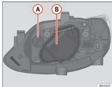
Fig. 156 Lámparas del faro AFS
